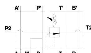
Cetop underplader med aflastningsventil
