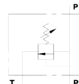
Trykbegrænsningsvent In-line montage
