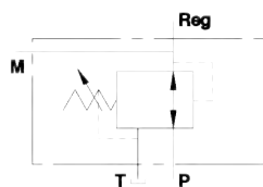
Direkte virkende trykreduktionsventil
