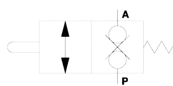
Endestopventil med knast, normalt lukket
