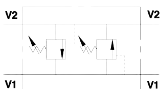
Dobbelt chockvent
