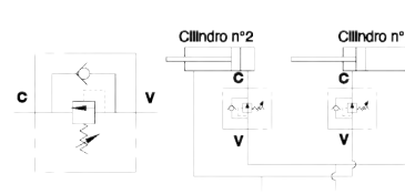
Direkte virkende sekvensvent
