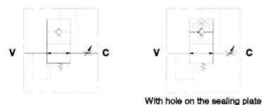
Slange sprængning ventil
