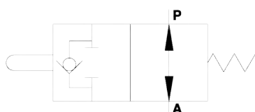
Trykknop-endeslagsventiler, normalt åbne med kontraventil
