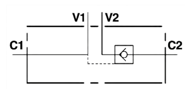
Pilotstyret kontravent
