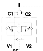
Dobbelt Overcenter vent for flange montage på Danfoss OMP/OMR
